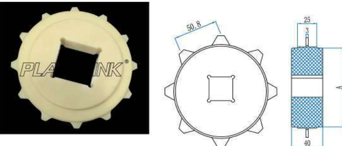
PL 620 链轮 PL 620 Sprocket
