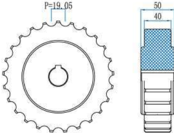
PL 812 系列 机加工主动链轮 PL 812 Series Machined driving sprocket
