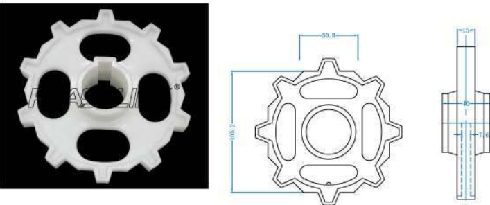
PL 620 链轮 PL 620 Sprocket
