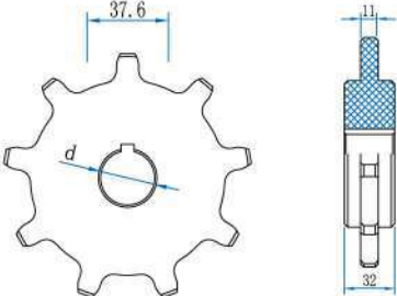
PL 83JC/103JC 系列 链轮 PL 83JC/103JC Series Machined driven sprocket
